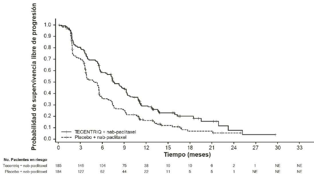
Figura 18: Curva Kaplan-Meier para la Supervivencia Libre de Progresión en pacientes con expresión PD-L1 \geq 1\% (IMpassion130)
