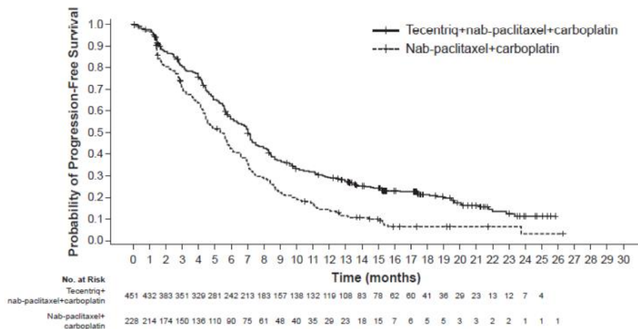
Figura 10: Curvas de Kaplan-Meier para supervivencia libre de progresión (IMpower130)
