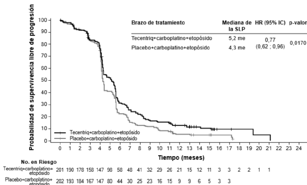
Figura 17: Curva Kaplan-Meier para la supervivencia libre de progresión (IMpower133)
