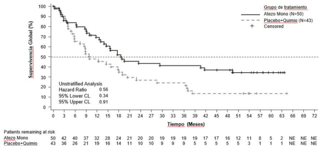
Figura 2 Kaplan-Meier Plot de Supervivencia Global en pacientes no aptos para recibir cisplatino cuyos tumores expresan PD-L1 alto (Grupo B vs. Grupo C)
