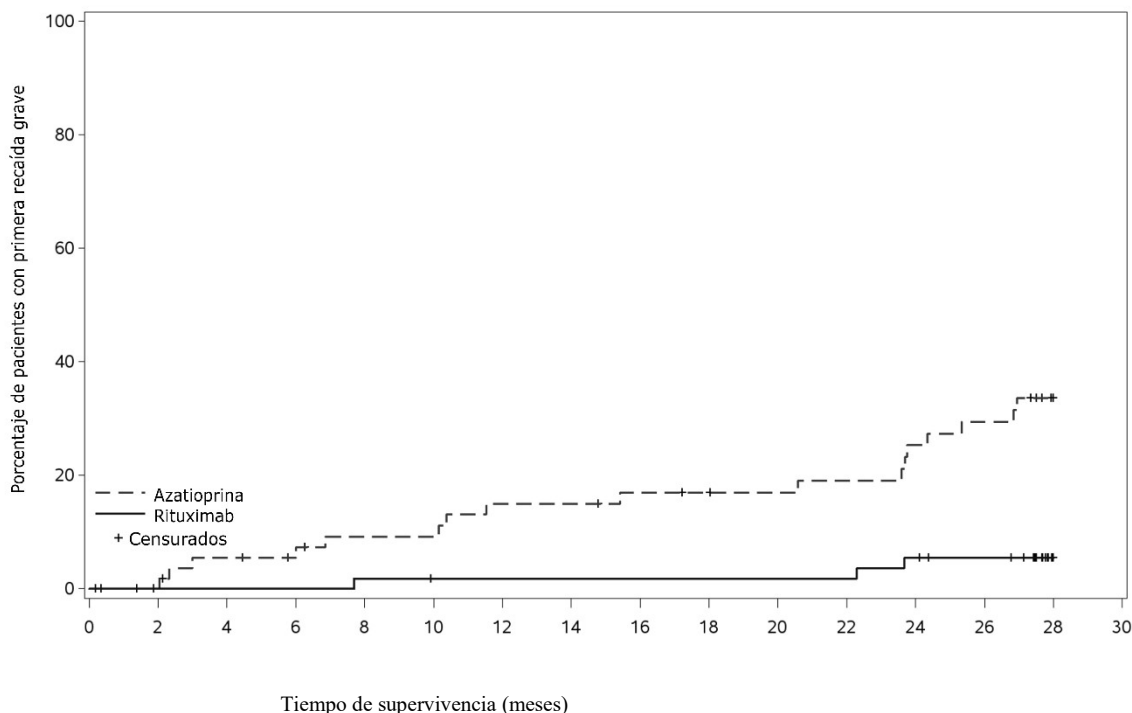
Figura 3: Curva de tasa de incidencia acumulativa del tiempo hasta la primera recaída grave.
