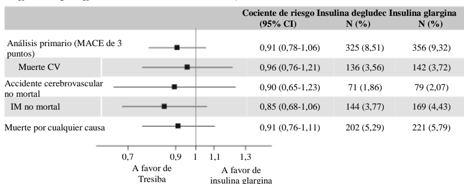
Figura 2 Diagrama de bosque del análisis de MACE combinados de 3 puntos y de los criterios de valoración individuales cardiovasculares en DEVOTE
